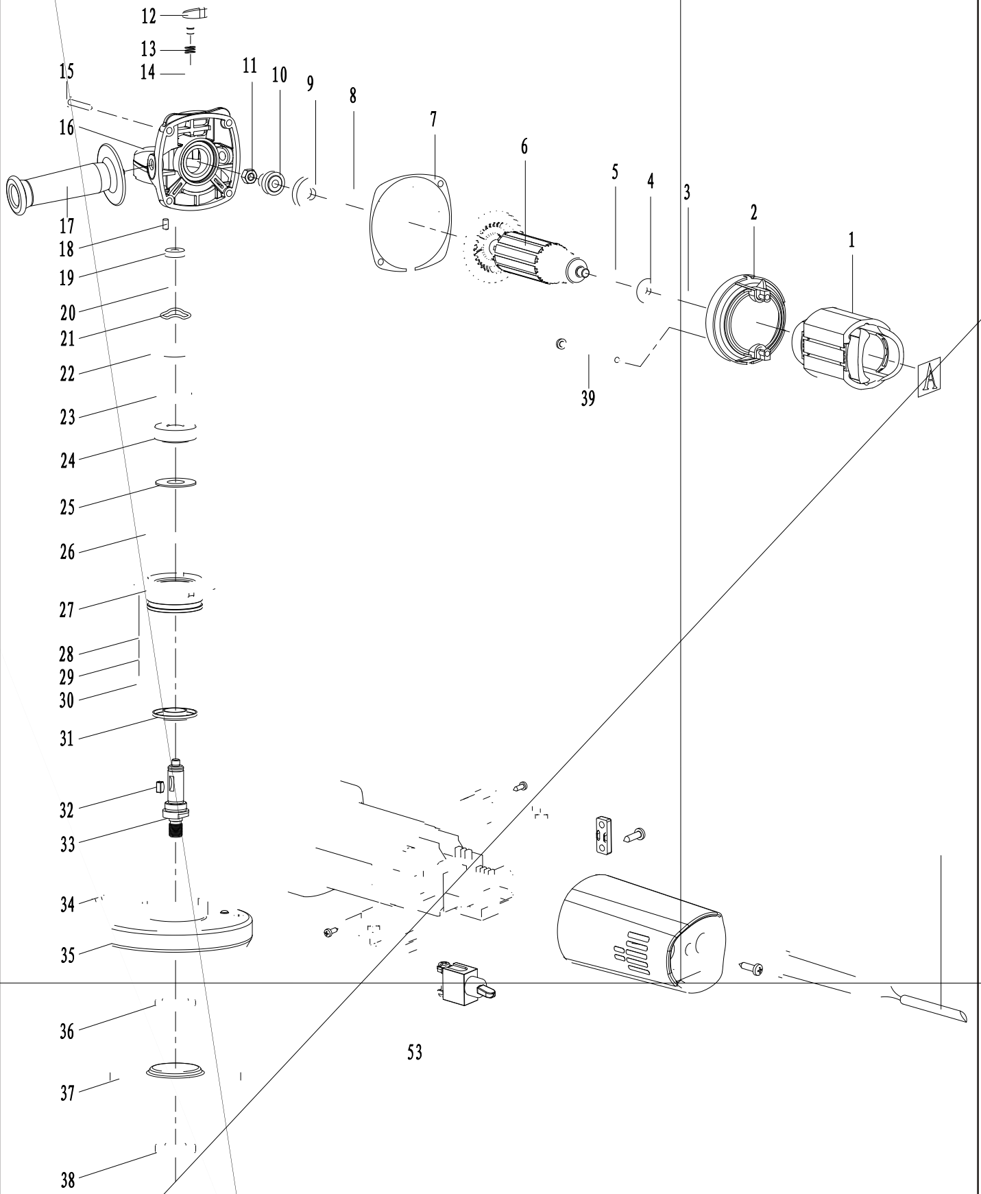
AG1005角向磨光机爆炸图
